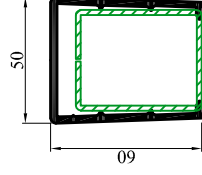
T6601 Profilé de renforcement extérieur - 560015 Renfort : T5117 - T5311 - T5319
