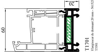
T1710 Elargisseur de dormant - 55x150 Renfort : T5002 - T5011
