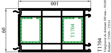
T1703 Elargisseur de dormant 60 mm - 561563 Renfort : T5309 - T5314
