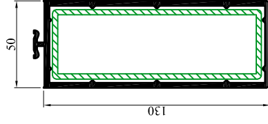
T6518 Profilé de renforcement - 627041 Renfort : T5303 - T5318
