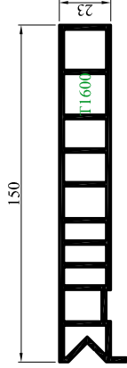
T1600 Tapée persienne de 150 x 23 - 560110
