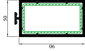
T6517 Profilé de renforcement - 627061 Renfort : T5307 - T5317 - T5322 - T5324
